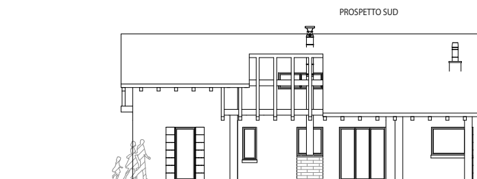
PROSPETTO SUD
