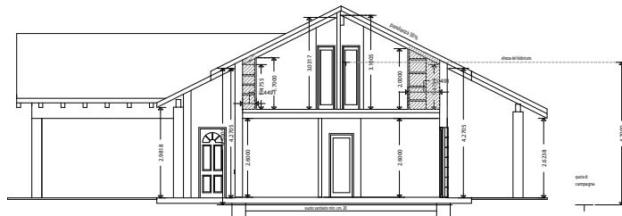
SEZIONE A-A
